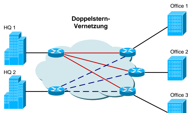
Abbildung 3: Doppelstern Topologie
