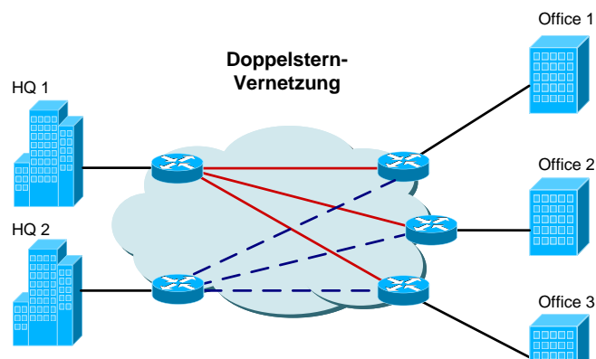
Abbildung 3: Doppelstern Topologie
